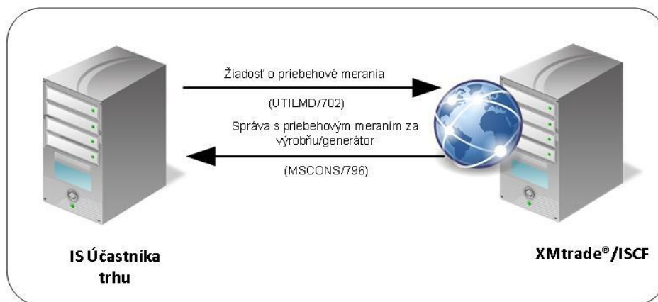
Obrázok 19 Rozhranie pre žiadosť o nepribehové merania výrobní/generátora
