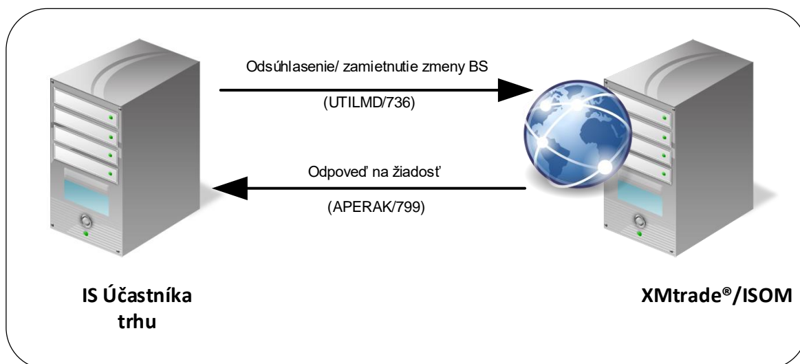
Obrázok 34 Rozhranie pre zamietnutie zmeny BS
